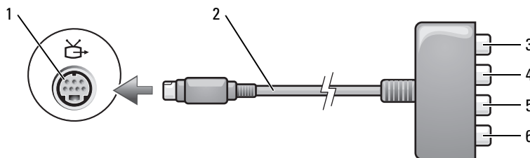
1 connecteur de sortie TV S-vidéo 2 adaptateur vidéo composante 3 connecteur audio numérique S/PDIF 4 connecteur de sortie vidéo composante Pr (rouge) 5 connecteur de sortie vidéo composante Pb (bleu) 6 connecteur de sortie vidéo composante Y (vert)
